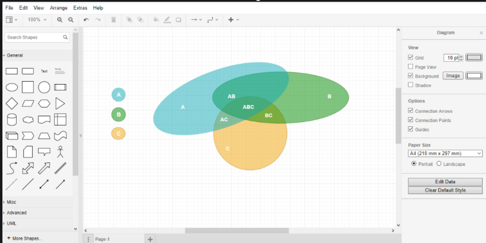
Venn Diagram
